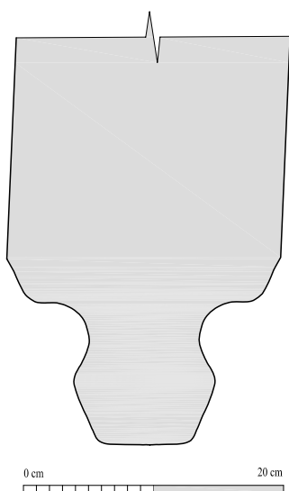
Obr. 3: Kostelec nad Vltavou, kostel Narození Panny Marie, profilace klebebního žebra severního ramene transeptu (sejmutí profilu F. Facincani, grafická úprava L. Beránková).
