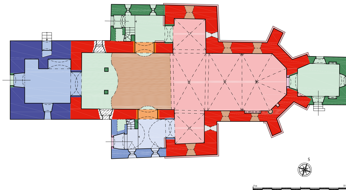
Obr. 7: Kostelec nad Vltavou, kostel Narození Panny Marie, půdorys přízemí. Orientační barevné vyhodnocení stavebního vývoje v novověku převzato z údajů publikovaných J. Adámkem a J. Varhaníkem v roce 2000. Šedivá – druhotně použitá okenní ostění ve východních zdích ramen transeptu, pocházející ze zbořeného románského kostela; červená – fáze z 1. pol. 14. století; fialová – druhotně osazené portály z 2. čtvrtiny 16. století; tmavě modrá – věž (1616); světle modrá – jižní kaple (1635); hnědá – zásahy z 2. pol. 17. století; zelená – přístavby ze 70. let 18. století; oranžová – probourání přízemních arkád v roce 1887; bílá se šrafkami – časově blíže nezařazené partie (zaměření F. Facincani, 2025; zaměření provedeno za použití laserového a skládacího metru; grafická úprava L. Beránková).
